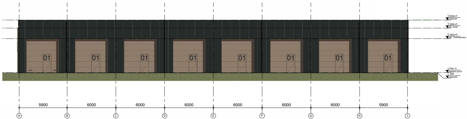
Rechtergevel B
