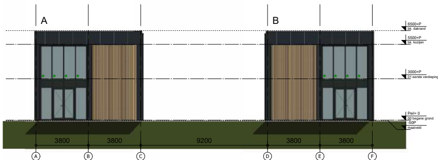
Voorgevel blok A en blok B
