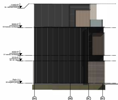
Linkergevel | Zuid-Oost
