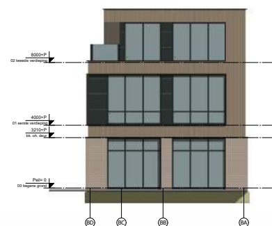
Rechtergevel | Noord-West
